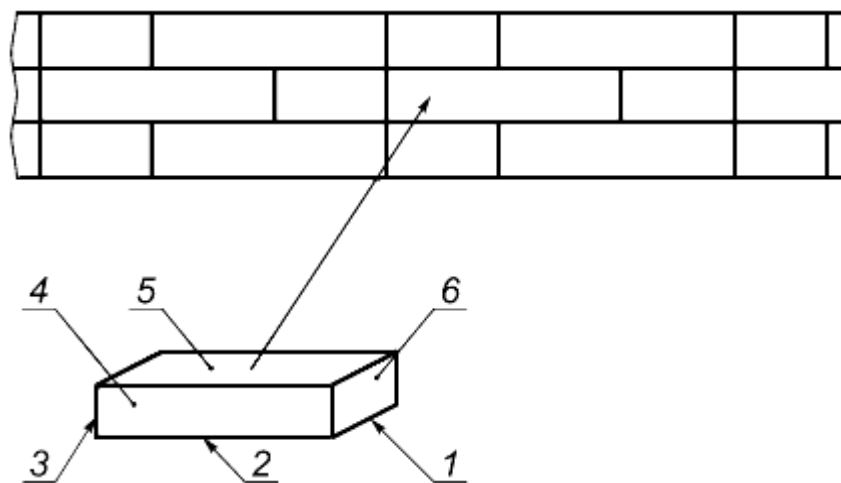
Рисунок 1 - Фрагмент кладки
